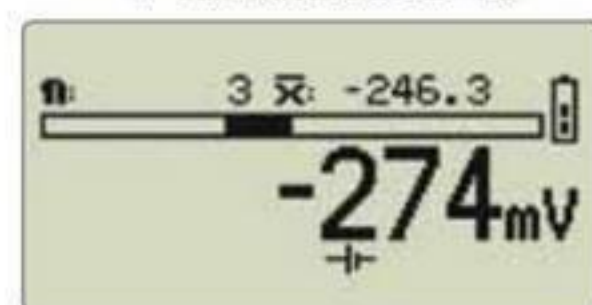
"半电池锈蚀模式显示
